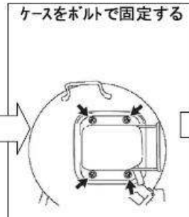
ケースの穴と、バルブ中心が一致するようにケースの位置を合わせる。
